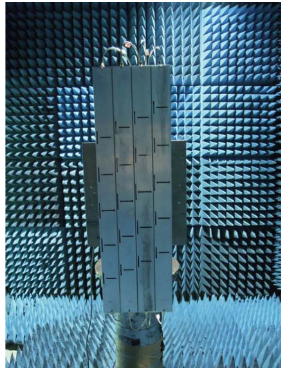
3.5GHz CP Slot Array Antenna
